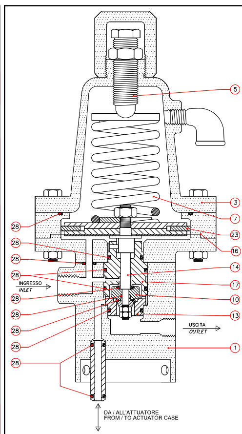
602 ON OFF SENZA PORTATA / NON FLOWING ON OFF
