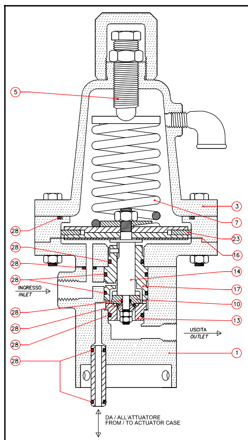
601 MODULANTE CON PORTATA / FLOWING MODULATING
